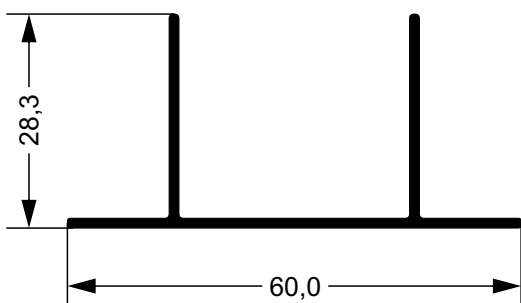
35015 C 0,401 kg/m Suporte Vertical Protetor Lateral
