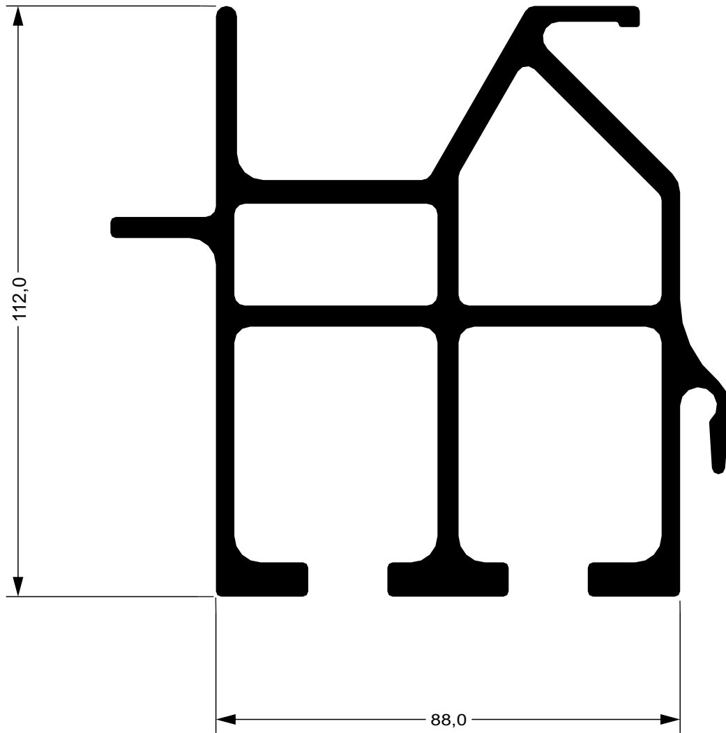
781433 E 6,497 kg/m Perfil Sider
