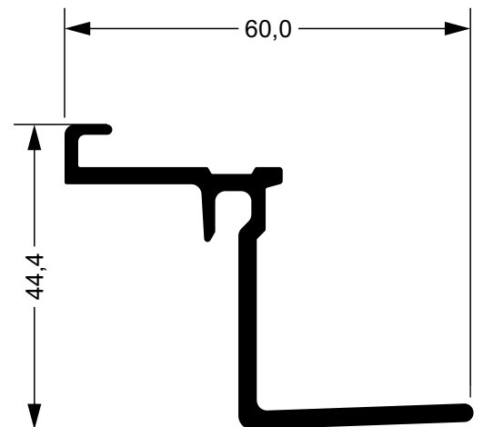
39685 0,797 kg/m Perfil Teto
