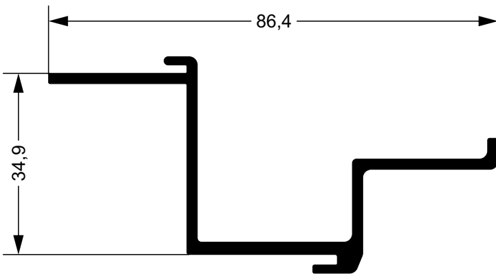
39577 0,886 kg/m Perfil Batente Porta
