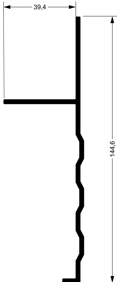
391187 C 1,314 kg/m Longarina Inferior
