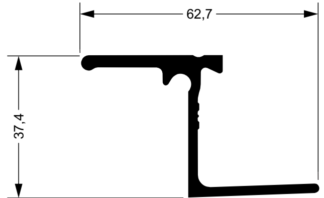
40005 0,852 kg/m Perfil Teto
