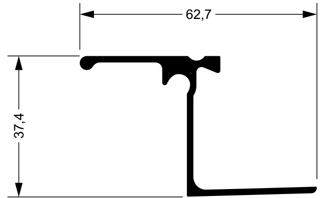
40007 0,700 kg/m Perfil Teto
