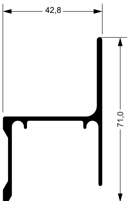
39314 0,886 kg/m Cadeirinha
