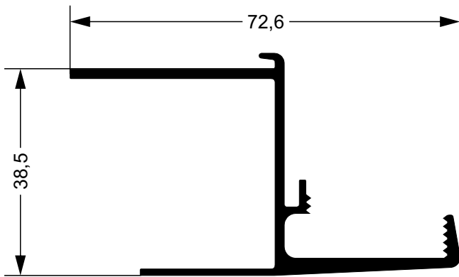
39340 0,870 kg/m Perfil Porta
