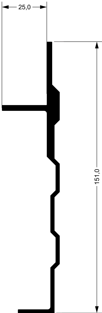
19364 1,712 kg/m Longarina Inferior
