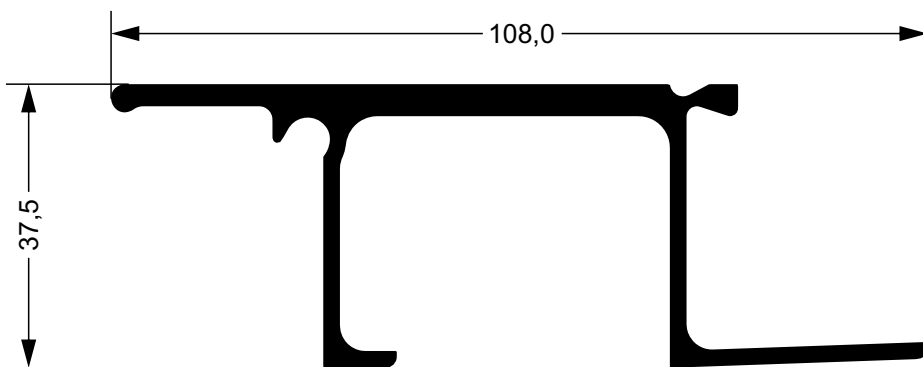
39173 1,681 kg/m Perfil Teto
