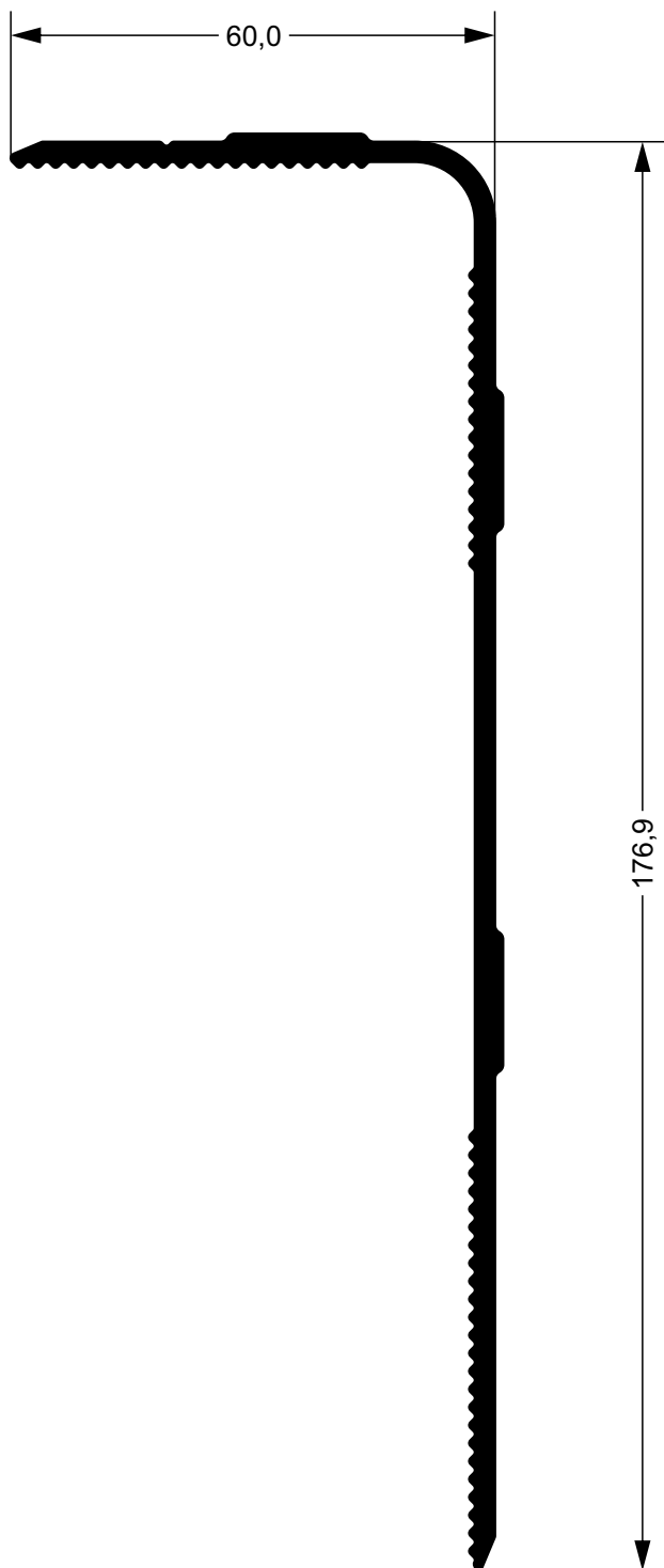
29274 D 1,811 kg/m Saia Externa Grande
