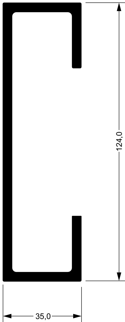
39102 2,560 kg/m Perfil C com Vinco
