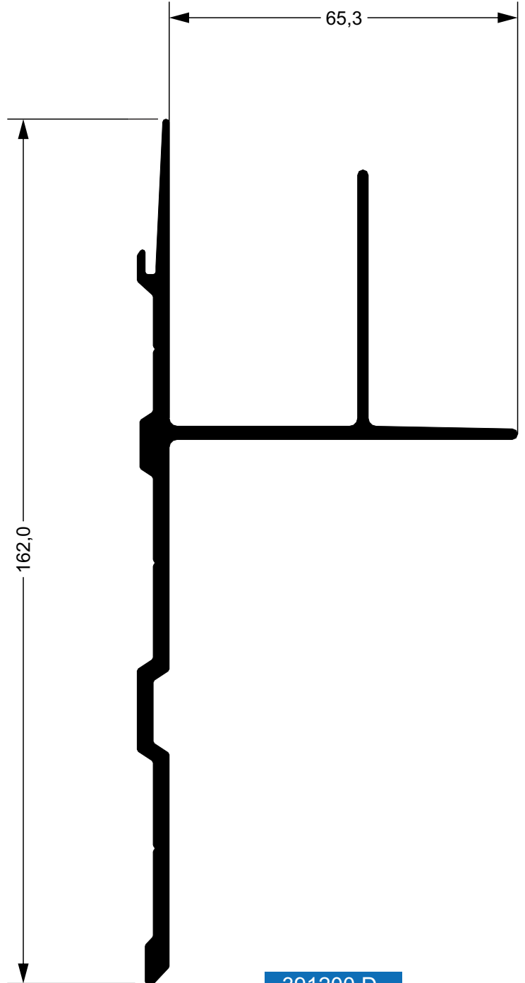
391200 D 2,073 kg/m Longarina
