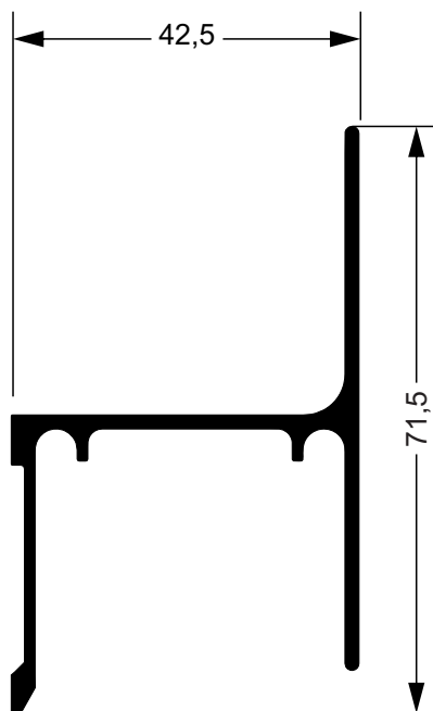
39177 0,816 kg/m Cadeirinha
