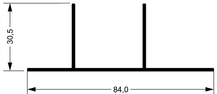
391613 C 0,538 kg/m Suporte Vertical Protetor Lateral
